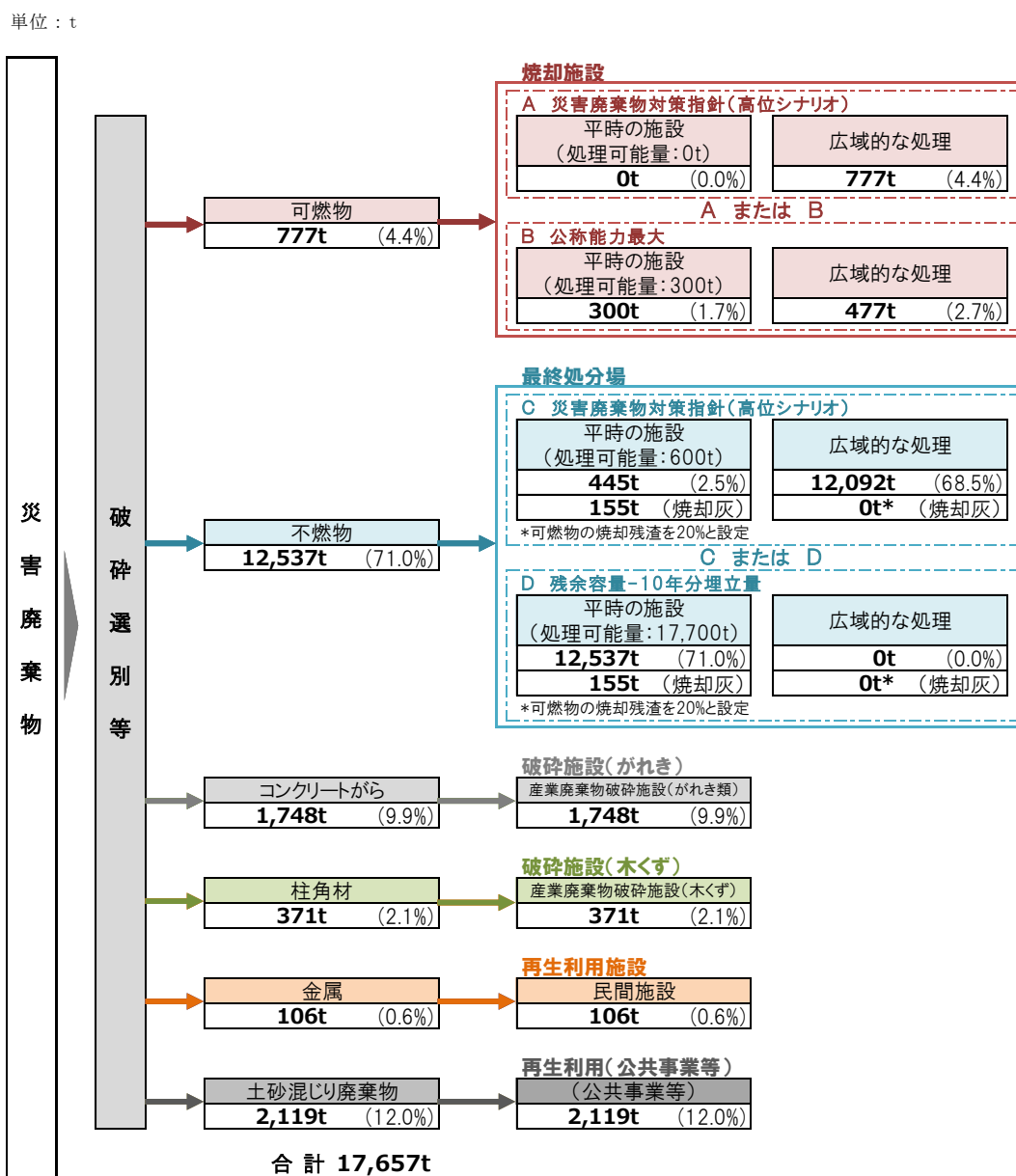
図 1 0 想定風水害発生における災害廃棄物処理フロー
