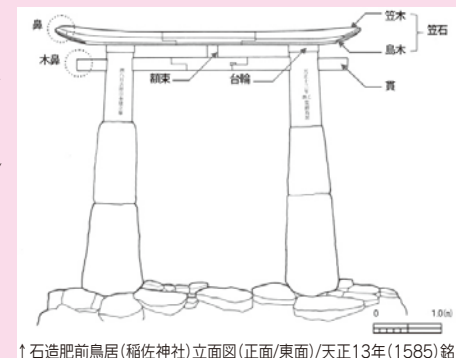
↑石造肥前鳥居(稲佐神社)立面図(正面/東面)/天正13年(1585)銘
