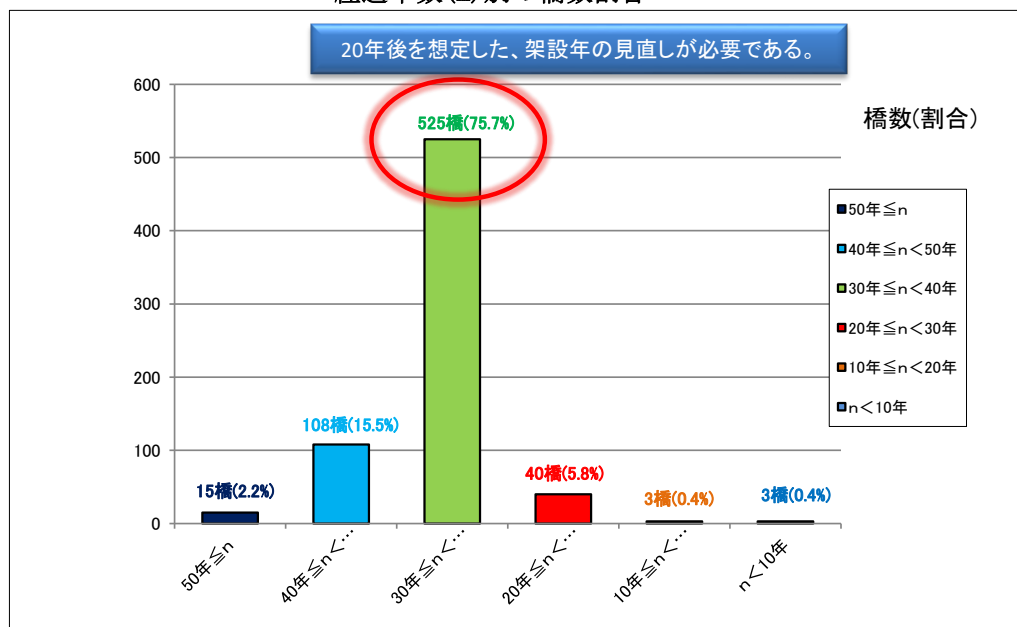
経過年数(n)別の橋数割合
