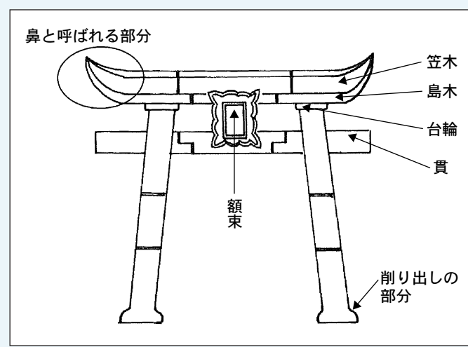
■肥前鳥居の名称 『肥前鹿島の石造文化』佐賀県鹿島市 昭和53年に掲載の図面を改編
